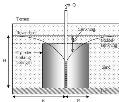
Figur 1: viser sænkning i et frit magasin. R_w angiver den påvirknings radius, mens R angiver radius af BNBO.
